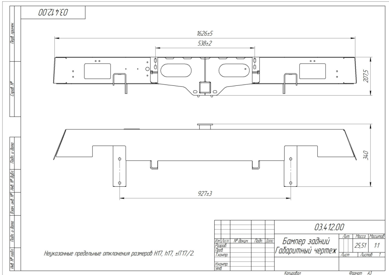
Рис. 3 Габаритный чертёж
