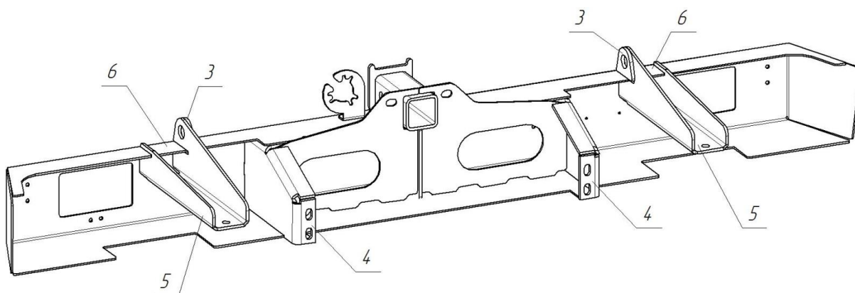
Рис.2 Бампер вид сзади (повёрнут)
