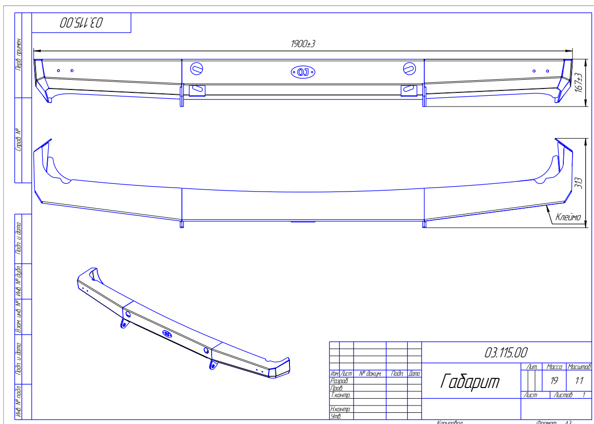
Рис. 3 Габаритный чертёж
